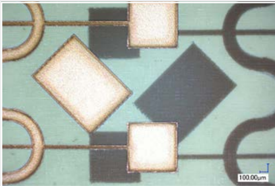
LPKF ProtoLaser R4 加工薄膜双面线路
