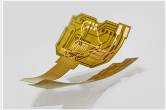
单、双面层压柔性电子材料的切割与电路图形制作 (DuPont Pyralux)
