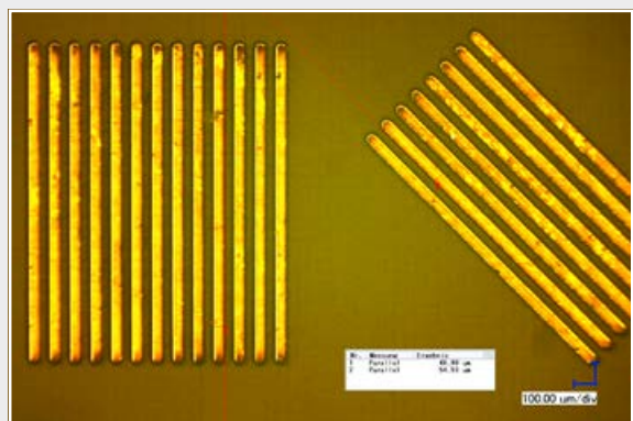
生物相容性材料如 LCP 和 COC, 表面薄膜电路层制作, 线宽小于 50 微米
