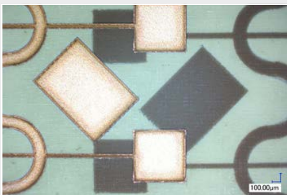
双面聚酰亚胺覆铜板, 9 微米铜箔, 基材厚度 25 微米
